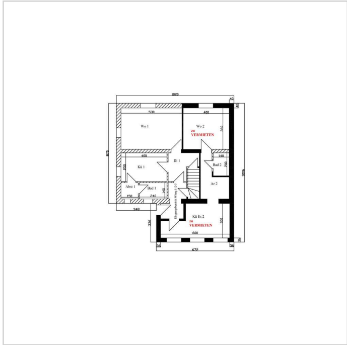
Grundrisse-EG
